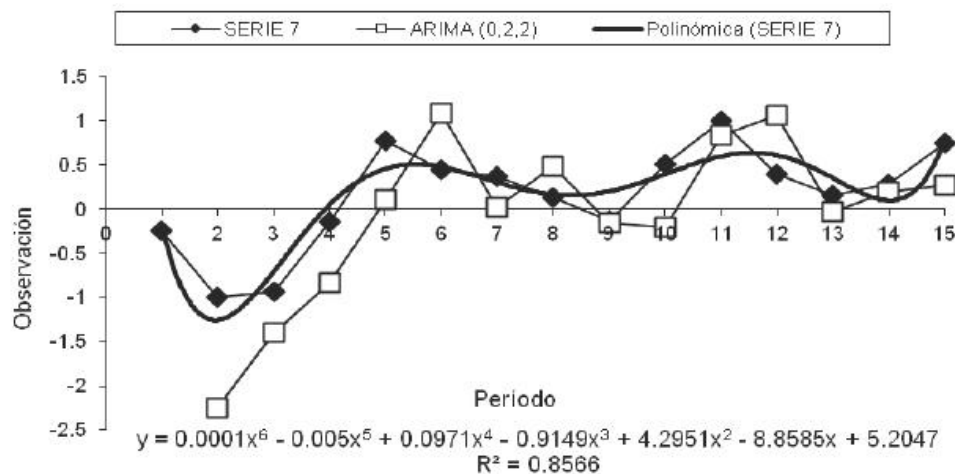
Figura 2. Serie de tiempo 7 vs. Pronóstico ARIMA (0, 2, 2).
